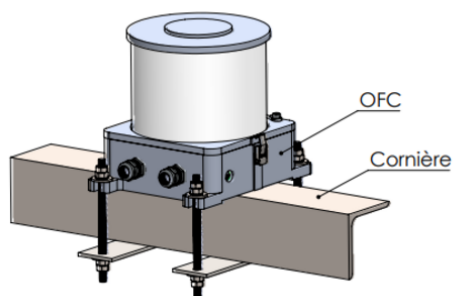
Potence de fixation pour cornière horizontale pour balise OFC
