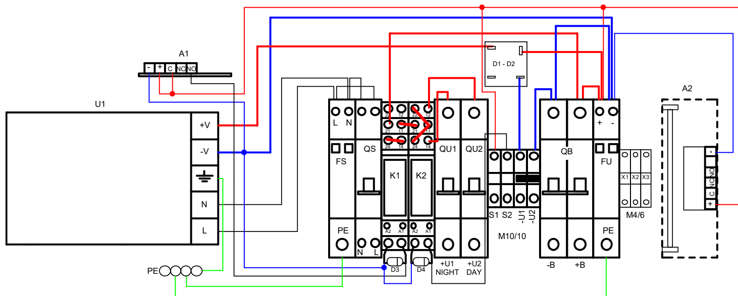
CABLAGÉ CONTACT NC
