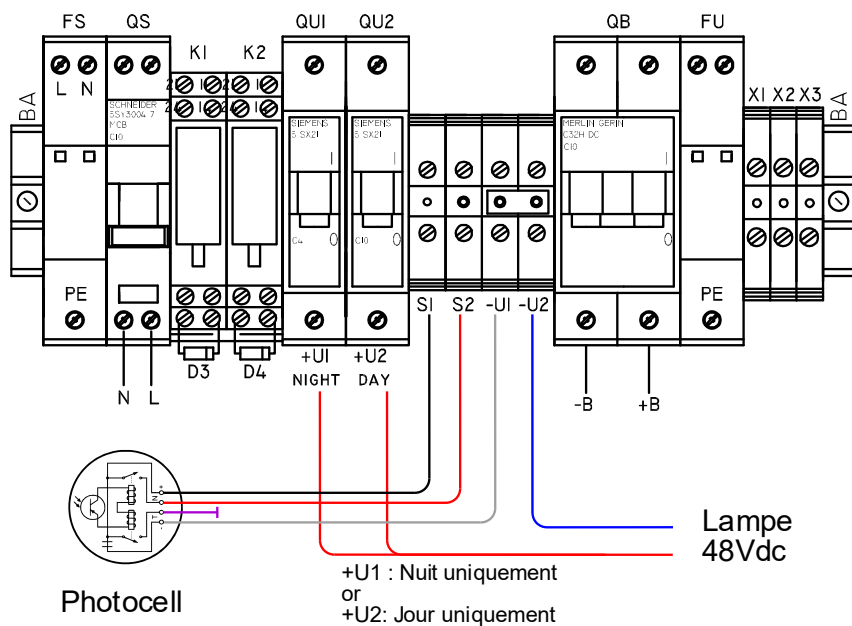
Branchement avec sonde crépusculaire
