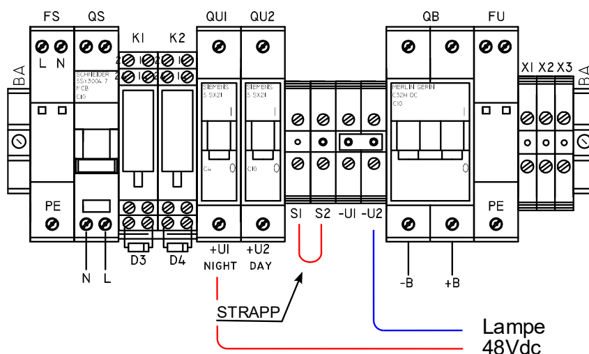
Branchement sans sonde crépusculaire
