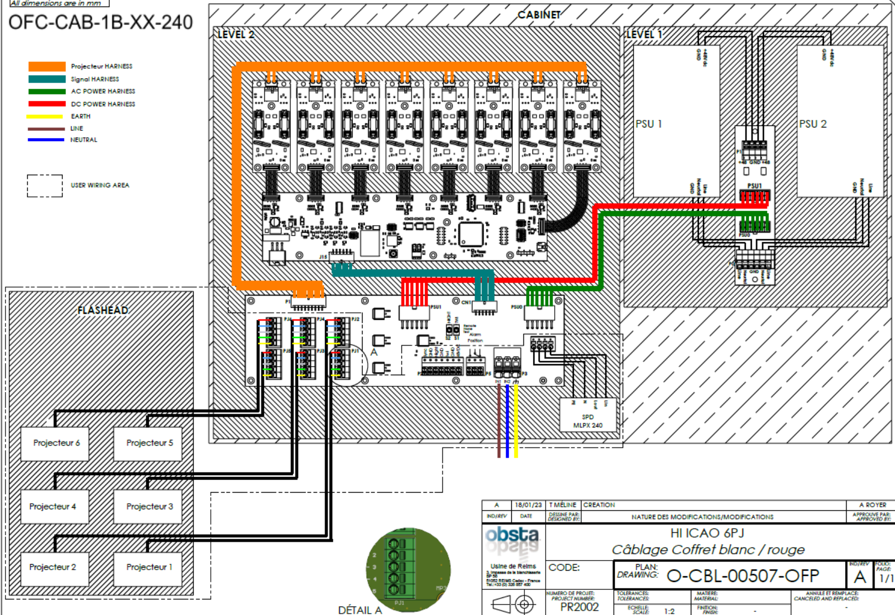
DÉTAIL A
