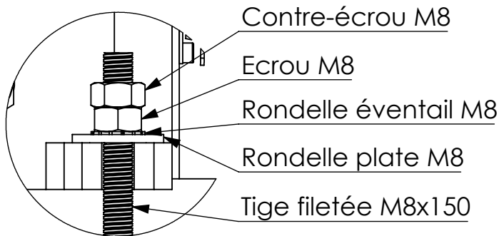
DÉTAIL A ECHELLE 2 : 3
