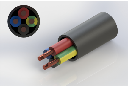
cablE 4G1,5
