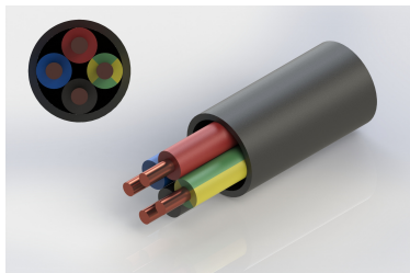
Câble 4G1,5 gaine PE
